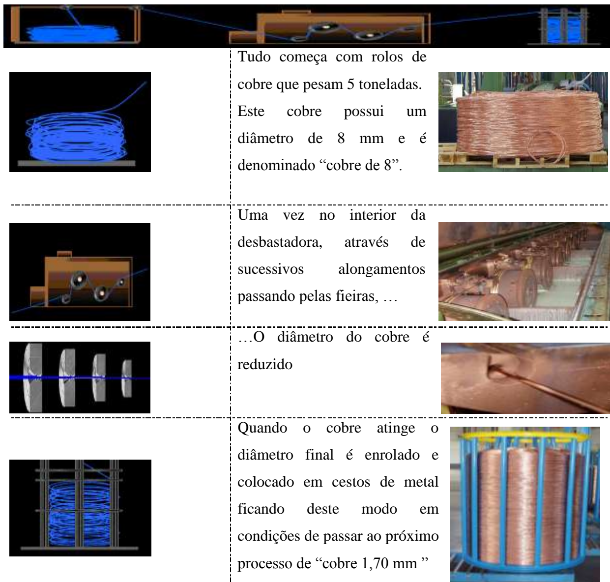
Figura 9: Processo de Debastagem
